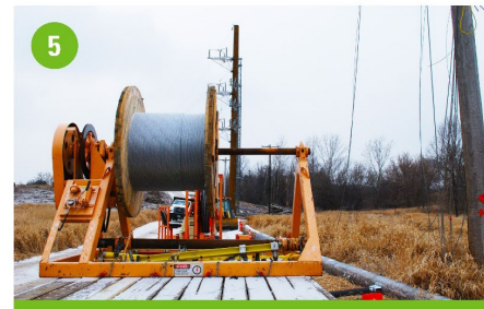
5 String wires
